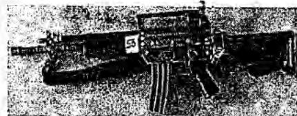
VISTA GENERAL Y MEDIANO ACERCAMIENTO DEL FUSIL CALIBRE 5.56X45 MM. NATO (.223), MARCA BERETTA, MODELO SCP 70/90, MANUFACTURA ITALIANA, SERIE [REDACTED]
